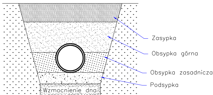
Rys 7 przekrój wykopu
